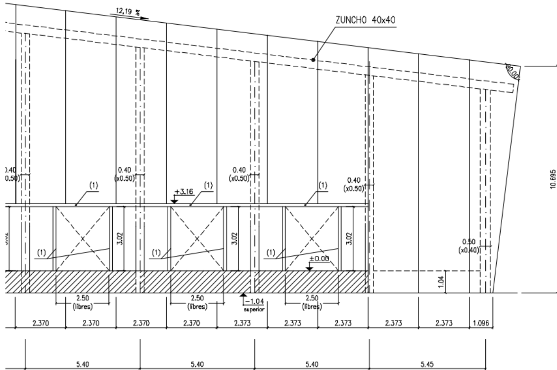
Medidas de la pared de Tavernes de la Valldigna
