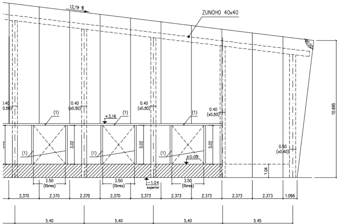
Mesures pared de Tavernes de la Valldigna.
